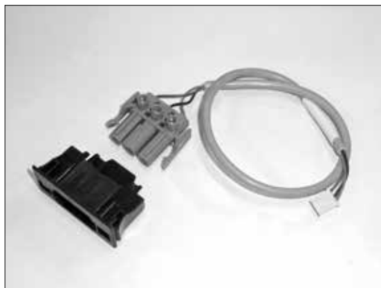
Kód: S0662 3-pinový konektor s kabelem pro připojení snímače otáček odtahového ventilátoru (UCJ4C82B) kotle D80P, P80
