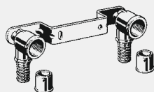
Montážní jednotka - Rp-závit Vybavení krátké koleno z červeného bronzu, držák (zalomený) z pozinkované oceli model 2724
