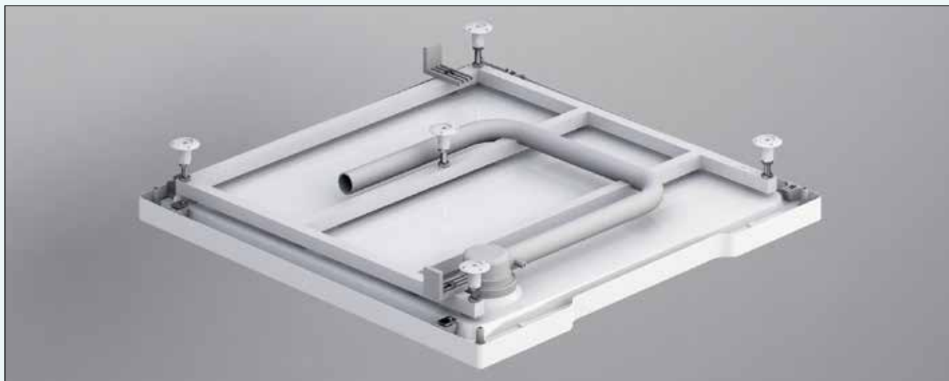
Čtvercová vanička (pohled na spodní stranu) se svařovaným rámem
