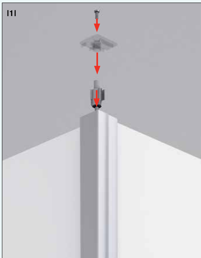
1. nerezová spojovací tyč umožňuje vertikální ukotvení profilů ve 3 rozích (zadní stěna – pohled zezadu – vrchní část)
