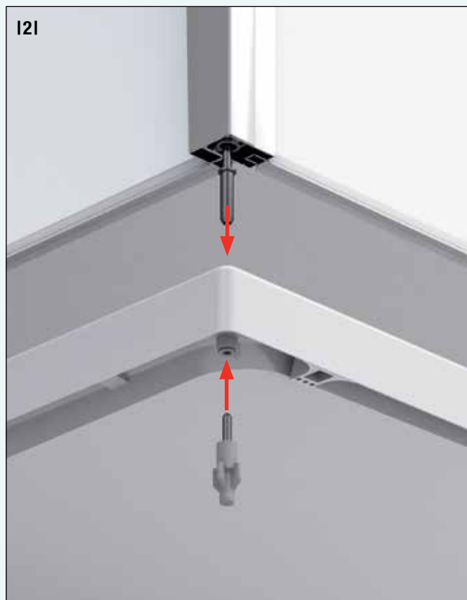
2. nerezová spojovací tyč (spojení s vaničkou – spodní část)
